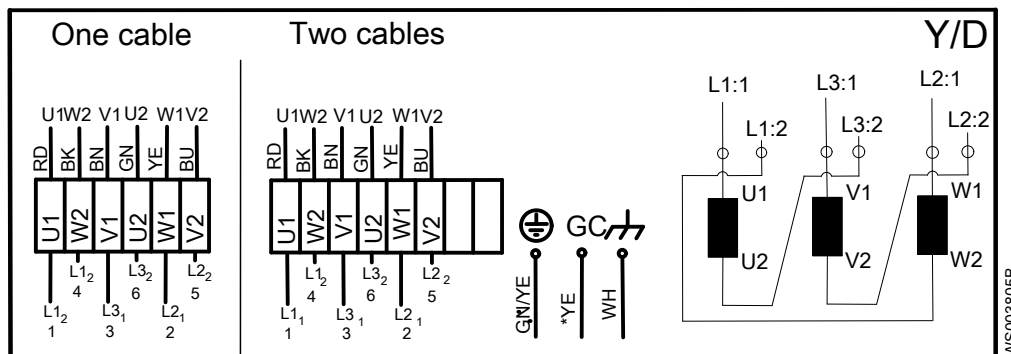
Рис. 12: «Звезда-треугольник»
