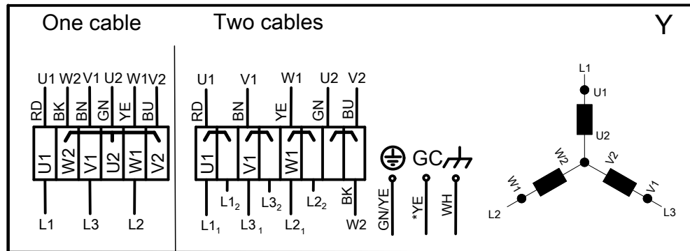
Рис. 10: Соединение «звезда»
