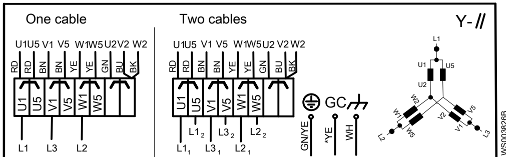
Рис. 13: Параллельное соединение звездой
