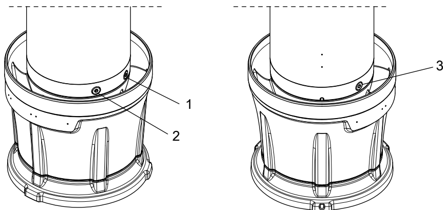
Рис. 23: С рубашкой охлаждения
