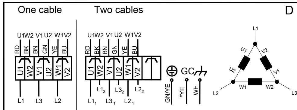
Рис. 11: Соединение «Треугольник»
